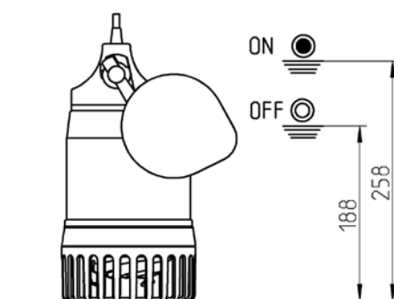
Afmetingen en schakelhoogtes spec. pompvlotter UV3 S (mm)
