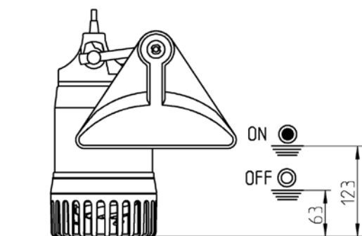
Afmetingen en schakelhoogtes spec. pompvlotter UV3 S (mm)
